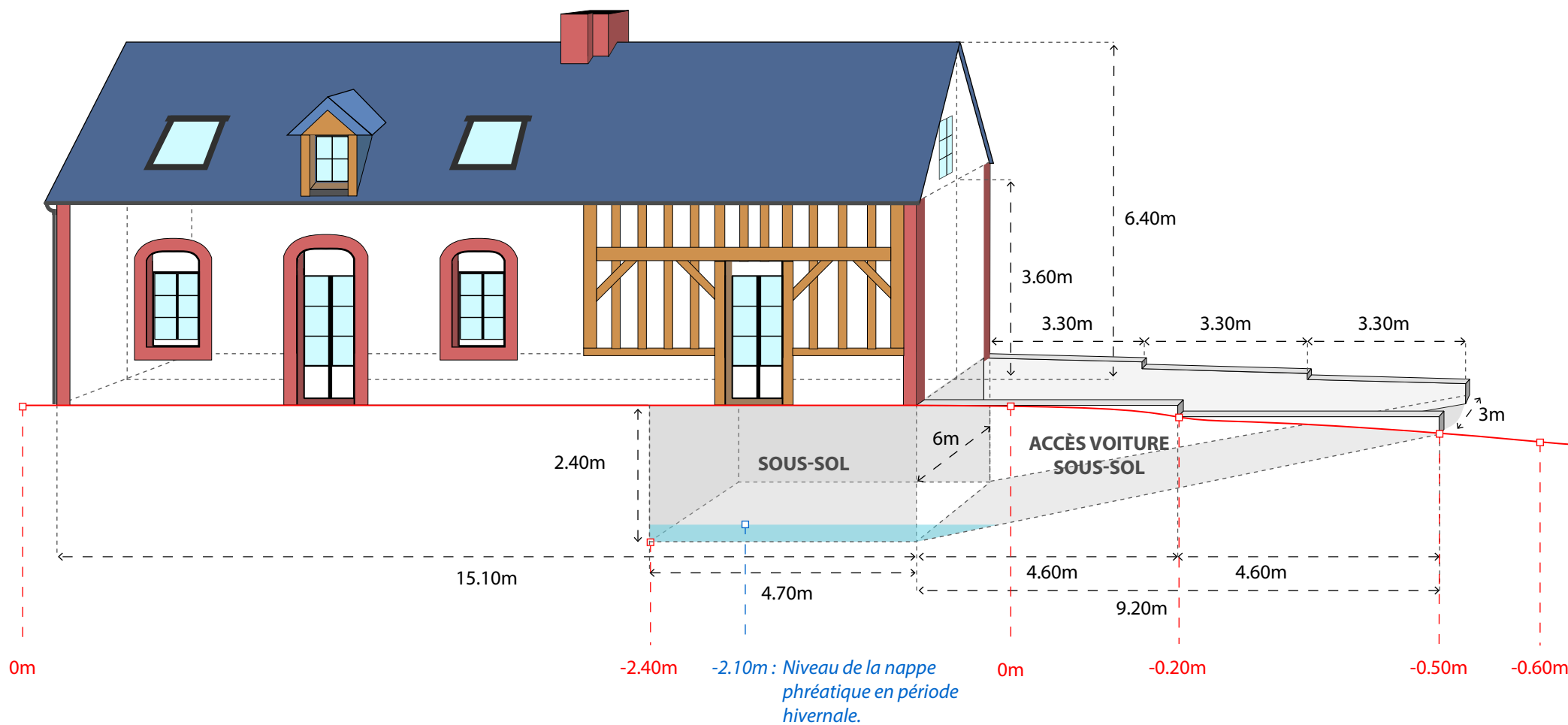
PLAN EN COUPE FACADE OUEST
